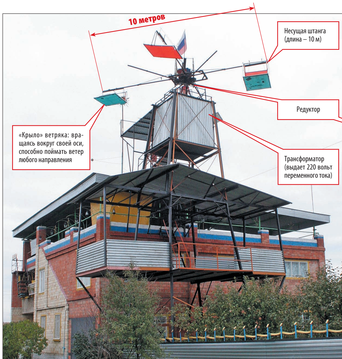
Ветряк, с помощью которого изобретатель Григорий Пономарев добывает электроэнергию, установлен прямо на его доме в Октябрьском поселке. Всю конструкцию туляк сделал сам.
