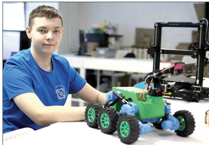
Володя Савин сделал машину с манипулятором, которая может быть полезна в чрезвычайных ситуациях.
