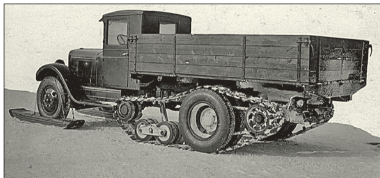
Грузовой вездеход ЗИС-33: к передним колёсам крепились специальные лыжи, на задние надевались съёмные полугусеницы.
