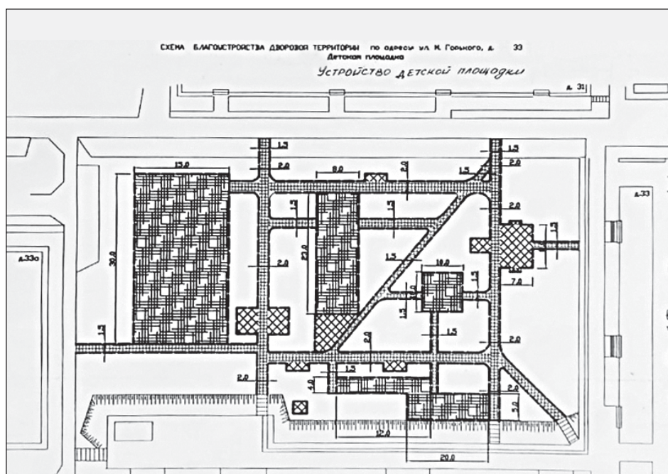
Схема обустройства детской площадки. Всё заштрихованное – либо асфальт, либо резина.
