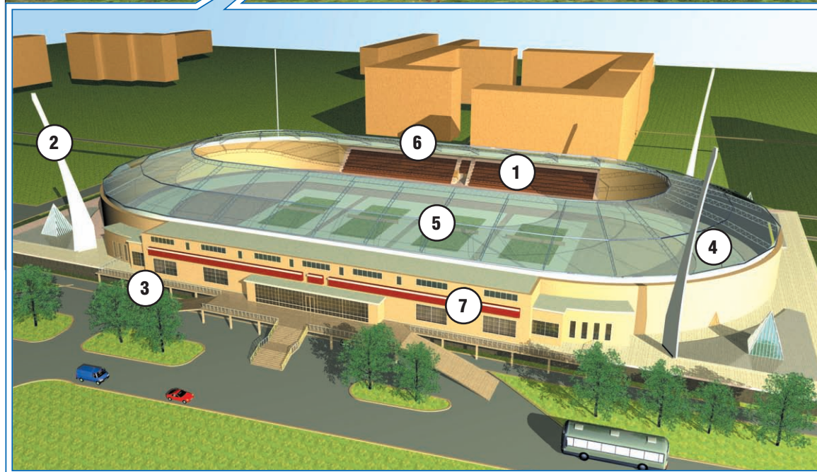
УСЛОВНЫЕ ОБОЗНАЧЕНИЯ: 1. Трибуны на 3000 человек. 2. Крепления для крыши. 3. Подземные гаражи. 4. Конькобежные дорожки. 5. 4 теннисных корта. 6. Гостиница для спортсменов под трибуной. 7. Раздевалки под трибуной.
