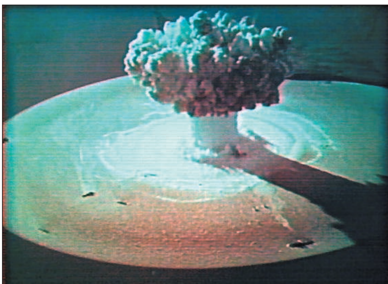
10 октября 1957 года, 10.00 по московскому времени, губа Черная: самый мощный подводный ядерный взрыв.
