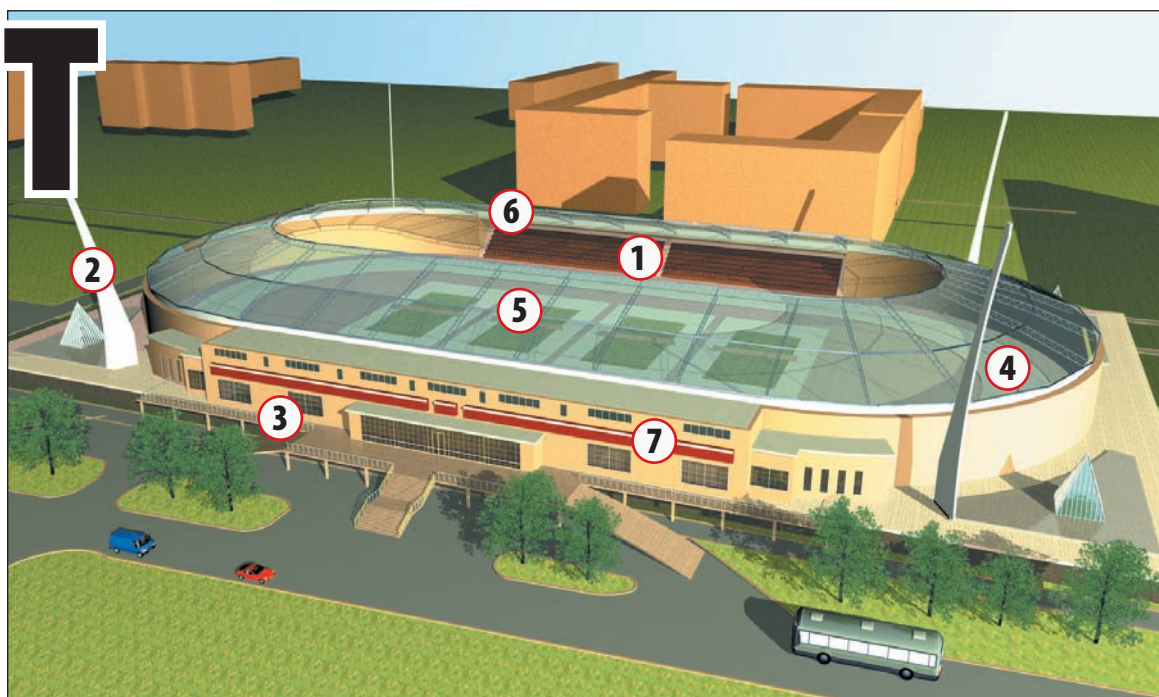
ПРОЕКТ КОНЬКОБЕЖНОГО ТРЕКА В ЗАРЕЧЬЕ: 1. Трибуны на 3000 человек. 2. Крепления для крыши. 3. Подземные гаражи. 4. Конькобежные дорожки. 5. 4 теннисных корта. 6. Гостиница для спортсменов под трибуной. 7. Раздевалки под трибуной.
