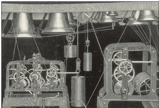
Схема башенных часов с курантами Торгового дома «Фридрих Винтер».
