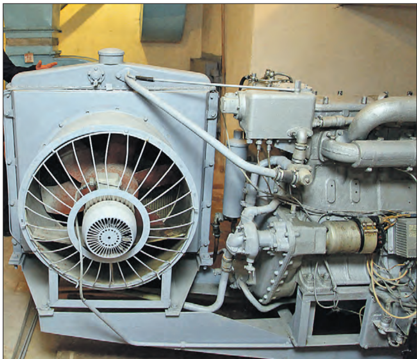
Большая комната отведена для дизельного генератора: в случае катастрофы он автономно обеспечит энергией всё убежище.
