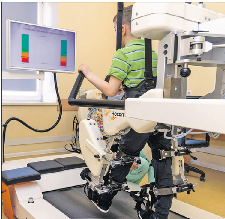
Центр оснащен роботизированным неврологическим и ортопедическим тренажером для восстановления навыков ходьбы - локоматом.
